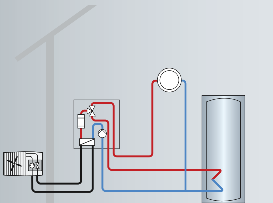
Vitocal 200-S unités intérieure et extérieure
